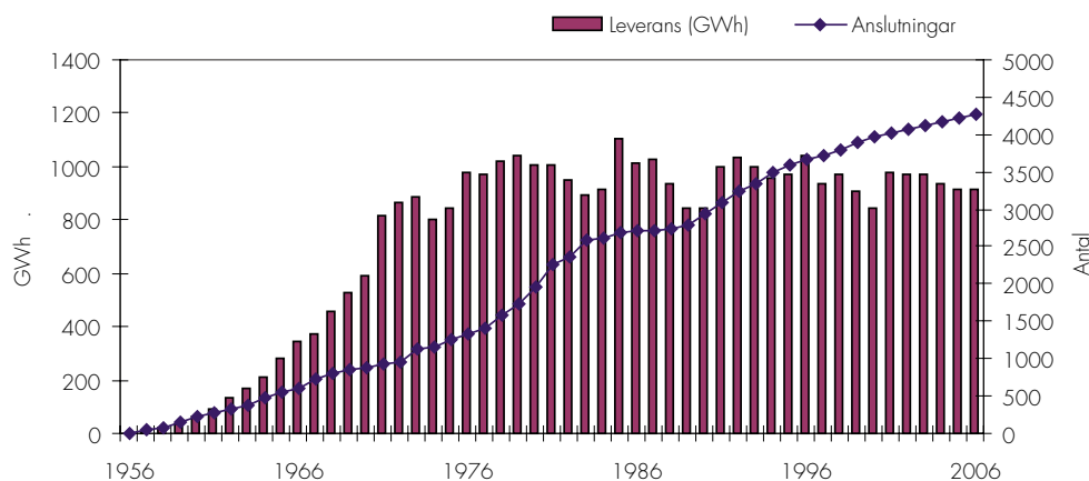
Figur 59. Fjärrvärmenätets utveckling i Örebro 1956-2006.
